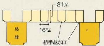
KM-1 [親子小組格縁]
